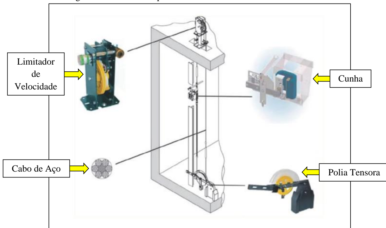
Figura 1 – Sistema completo de limitador de velocidade de elevadores
