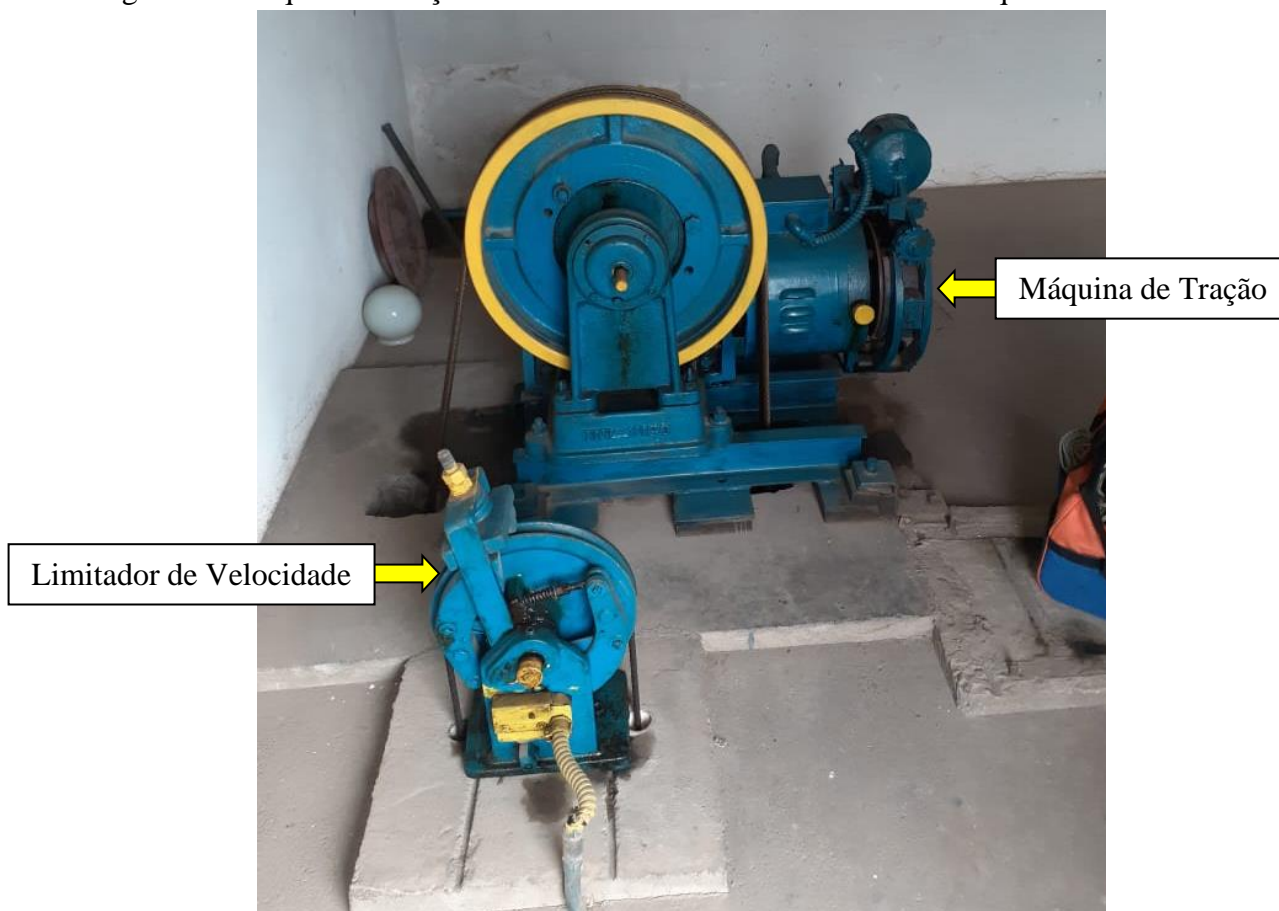
Figura 2 – Máquina de tração e limitador de velocidade na casa de máquinas de elevadores:
