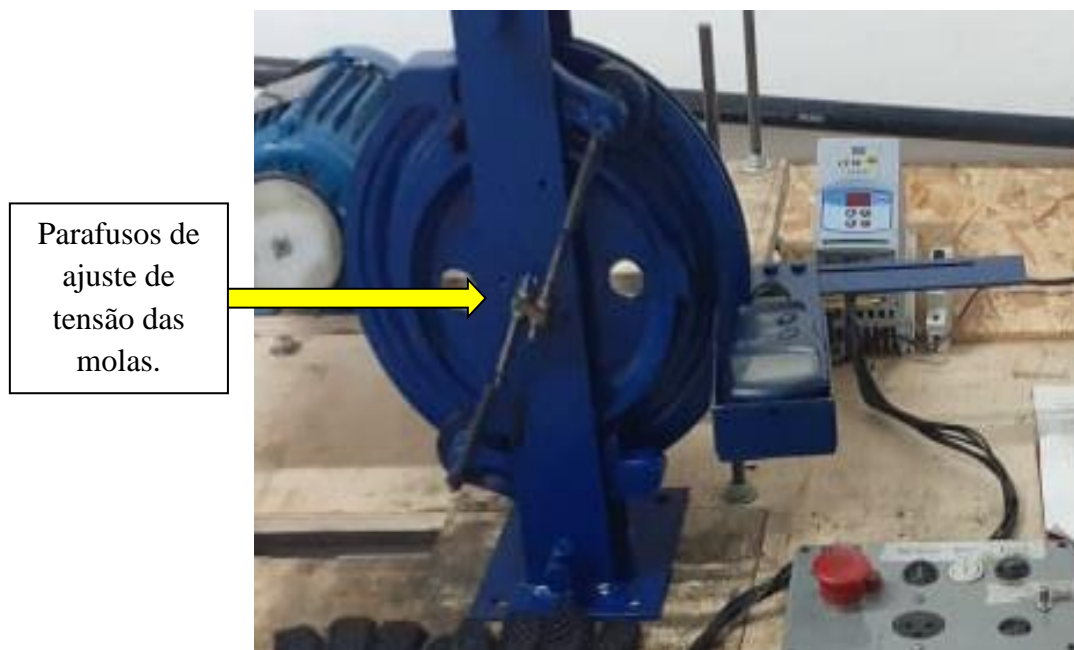
Figura 10 – limitador de velocidade sendo preparado para teste de bancada:
